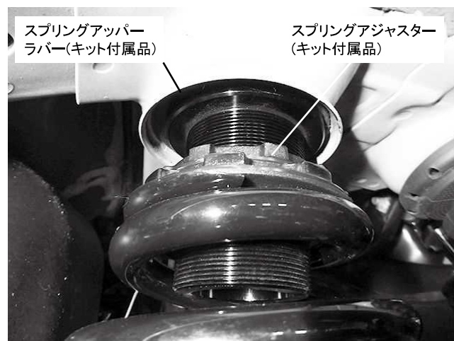
リアスプリング取り付け状態 ※スプリングアジャスター取り付けの際、アジャスター上部に キット付属スプリングアッパーラバーを取り付けてください ※純正アッパーラバーは取り外してください
