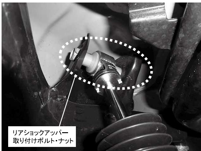
リアショックアッパー 取り付けボルト・ナット 1カ所締め付け 締め付けトルク: 120N・m(12.0kgf・m)
