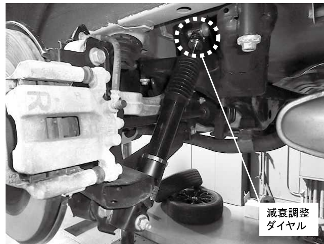
リアショックアブソーバー取り付け状態 ※減衰調整ダイヤルは構造上 リアショック上部にあります
