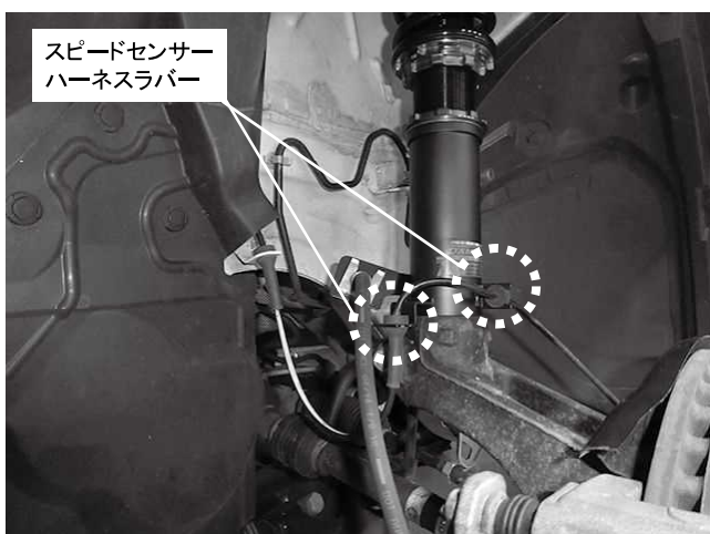
スピードセンサーハーネススラバー 2カ所取り付け ※スピードセンサーハーネスが突っ張っていたり しないか確認してください
