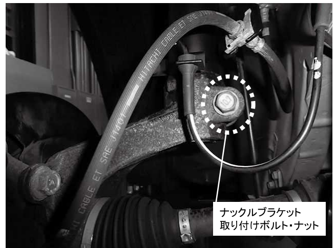
ナックルブラケット取り付けボルト・ナット 1カ所締め付け 締め付けトルク: 90N・m(9.2kgf・m)
