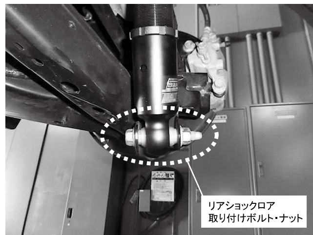
リアショックロア 取り付けボルト・ナット 1カ所締め付け 締め付けトルク: 120N・m(12.0kgf・m)
