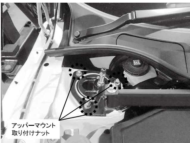
アッパーマウント 取り付けナット アッパーマウント取り付けナット 3ヵ所締め付け 締め付けトルク: 44N・m(4.5kgf・m) ※製品付属のM10ナットを使用してください
