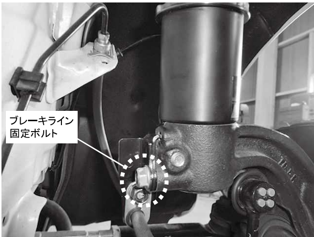
ブレーキライン 固定ボルト ブレーキライン固定ボルト 1ヵ所締め付け 締め付けトルク: 22N・m(2.2kgf・m)
