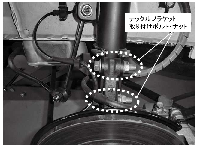
ナックルブラケット取り付けボルト・ナット 2カ所締め付け 締め付けトルク: 64N・m(6.5kgf・m)
