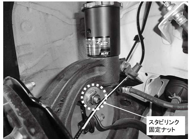
スタビリンク 固定ナット スタビリンク固定ナット 1ヵ所締め付け 締め付けトルク: 79N・m(8.1kgf・m)
