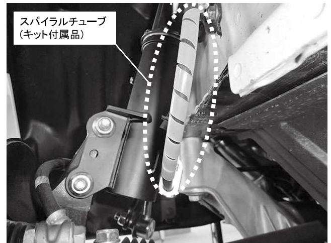
車両構造上ブレーキホースとボディとの クリアランスが狭くなります 同梱のスパイラルチューブを巻いて保護してください
