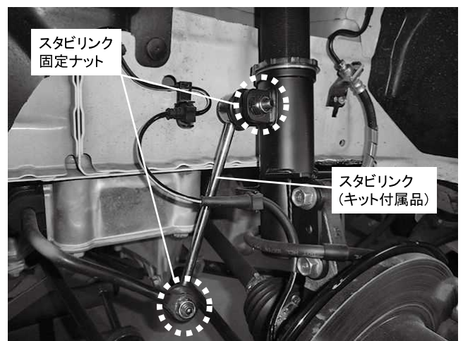
スタビリンク固定ナット 2カ所締め付け 締め付けトルク: 44N・m(4.5kgf・m)
