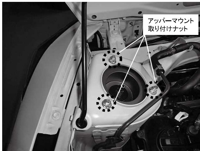
アッパーマウント取り付けナット 3カ所締め付け 締め付けトルク: 49\text{N}\cdot\text{m} ( 5.0\text{kgf}\cdot\text{m} ) ※製品付属のM10ナットを使用してください
