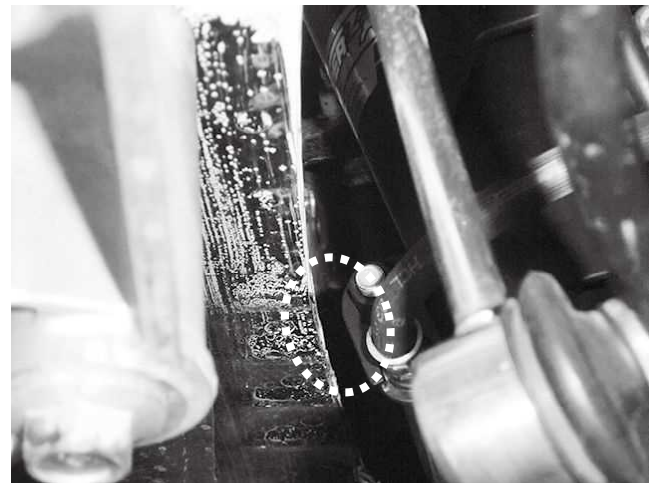
車両構造上ブレーキライン固定ステーと ボディとのクリアランスが狭くなります 干渉がないか確認してください
