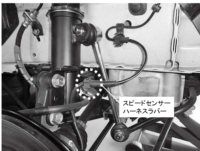
スピードセンサーハーネスラバー固定 ※ハーネスラバーがブラケットに固定できない、またはハーネスが 突っ張ってしまう場合には潤滑油を使用しラバーの位置を ハーネスの上部にずらして固定してください
