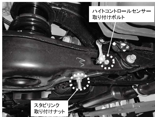
スタビリンク取り付けナット 1カ所締め付け 締め付けトルク: 30N・m(3.1kgf・m) ハイトコントロールセンサー取り付けボルト(左側のみ) 1カ所締め付け 締め付けトルク: 8.0N・m(0.8kgf・m)
