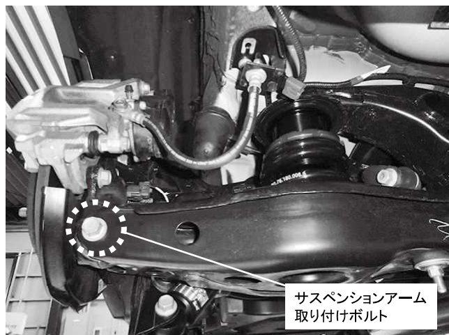
サスペンションアーム 取り付けボルト 1カ所締め付け 締め付けトルク: 90N・m(9.2kgf・m)
