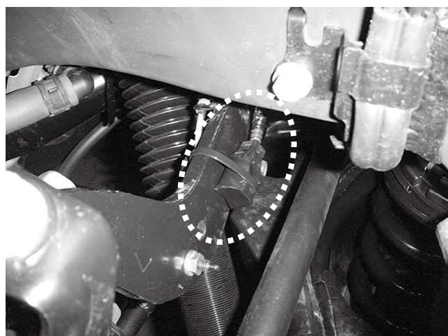
AVS装着車は純正ショックより取り外した コネクター・ハーネス類を走行時に干渉など しないようにまとめるなど保護してください
