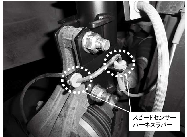
スピードセンサーハーネスラバー 2カ所取り付け ※スピードセンサーハーネスが突っ張ってたり しないか確認してください
