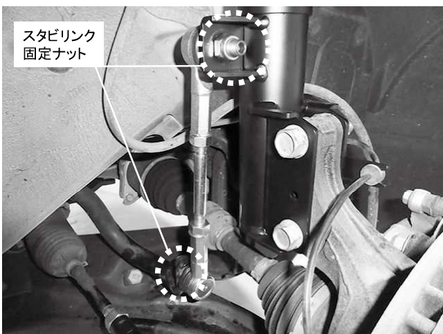
スタビリンク固定ナット 2カ所締め付け
