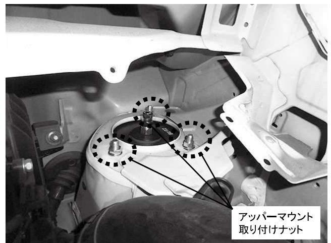
アッパーマウント取り付けナット
