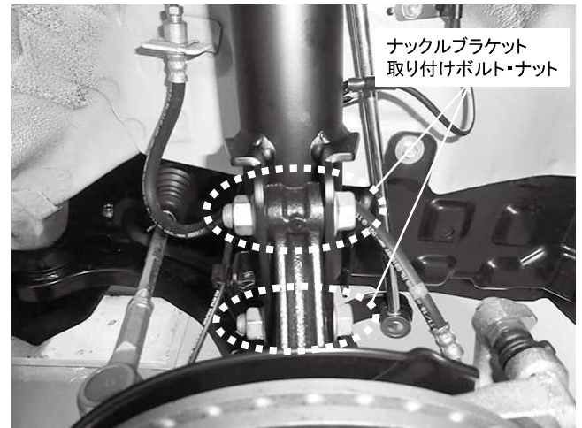
ナックルブラケット取り付けボルト・ナット 2カ所締め付け 締め付けトルク: 108N・m(10.9kgf・m)
