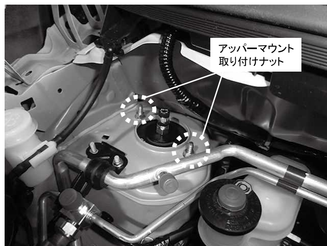
アッパーマウント取り付けナット 2ヵ所締め付け 締め付けトルク: 44\text{N}\cdot\text{m} ( 4.4\text{kgf}\cdot\text{m} ) ※製品付属のM8ナットを使用してください
