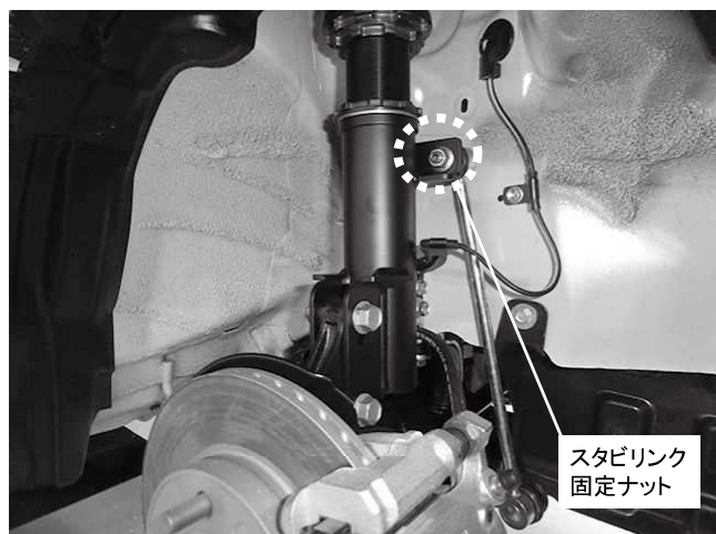
スタビリンク固定ナット 1ヵ所締め付け 締め付けトルク: 48\text{N}\cdot\text{m} ( 4.9\text{kgf}\cdot\text{m} )
