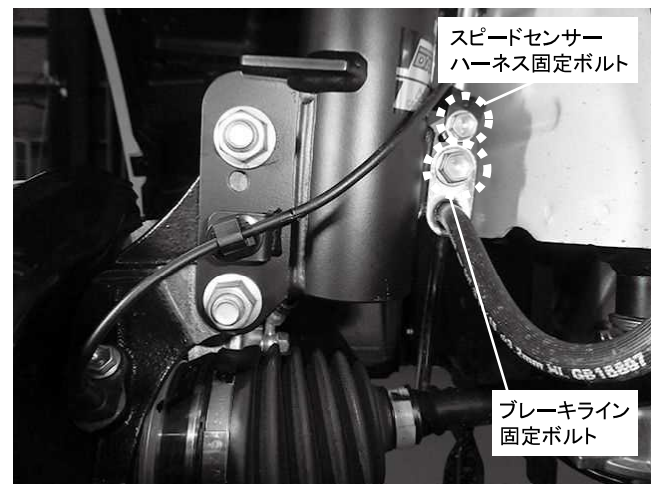
ブレーキライン固定ボルト 1カ所締め付け 締め付けトルク: 24.5N・m(2.5kgf・m) スピードセンサーハーネス固定ボルト 1カ所締め付け 締め付けトルク: 9.8N・m(1.0kgf・m)
