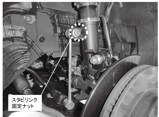
スタビリンク固定ナット 1カ所締め付け 締め付けトルク: 74N・m(7.5kgf・m) ※純正スタビリンクを使用してください
