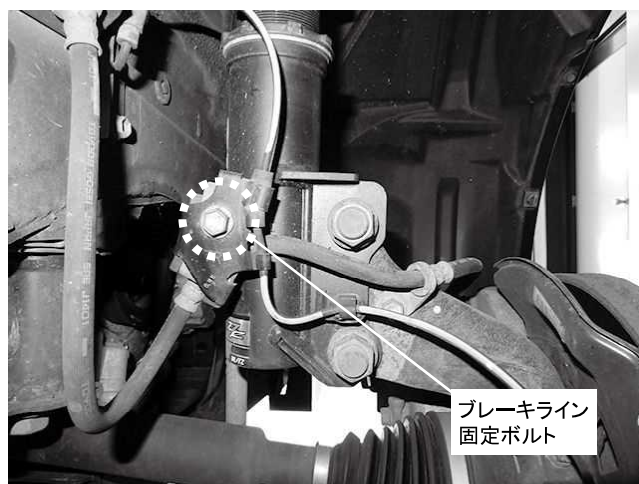
ブレーキライン固定ボルト 1カ所締め付け 締め付けトルク: 19N・m(1.9kgf・m) ※ネジ部に塗装がついて締め付けが渋い場合があります ※スピードセンサーハーネスと共締めしてあります
