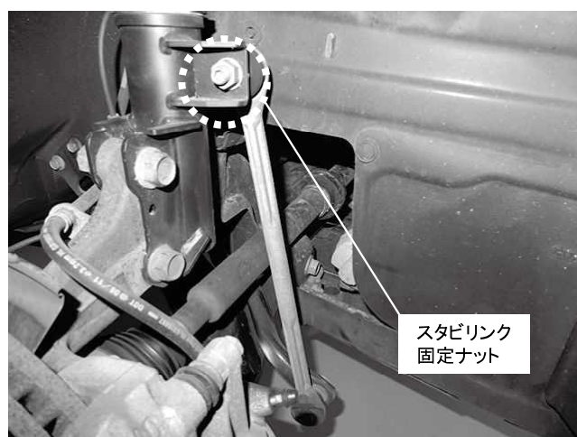
スタビリンク固定ナット 1カ所締め付け 締め付けトルク: 74N・m(7.5kgf・m)
