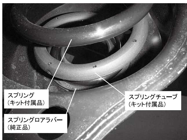
リアスプリング取り付け状態(下側) ※スプリングをサスペンションアームに取り付けの際、 純正スプリングラバーを取り付けてください ※スプリングが線間密着する際、必要に応じてスプリング チューブを使用してください
