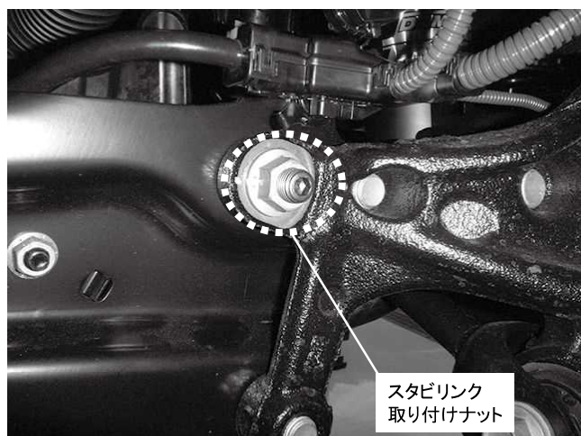
スタビリンク取り付けナット(上側) 1カ所締め付け 締め付けトルク: 75N・m(7.6kgf・m)
