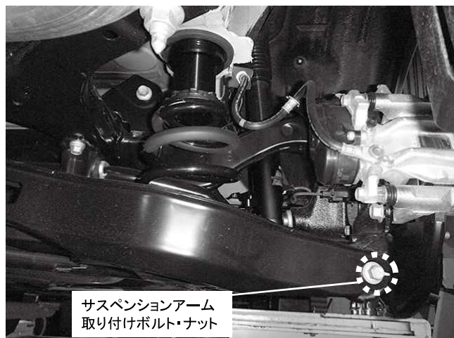
サスペンションアーム取り付けボルト・ナット 1カ所締め付け 締め付けトルク: 73N・m(7.4kgf・m)
