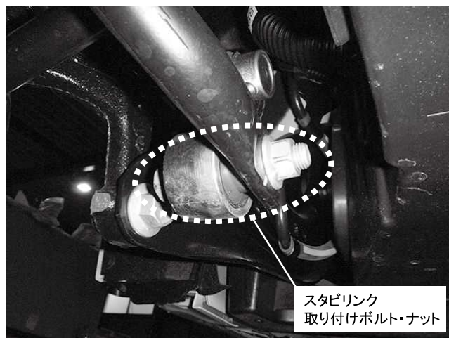
スタビリンク取り付けボルト・ナット(下側) 1カ所締め付け 締め付けトルク: 75N・m(7.6kgf・m)
