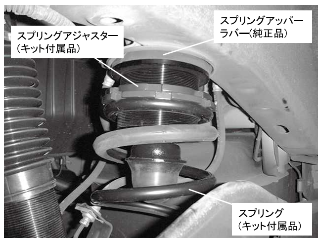
スプリングアッパ側取り付け状態
