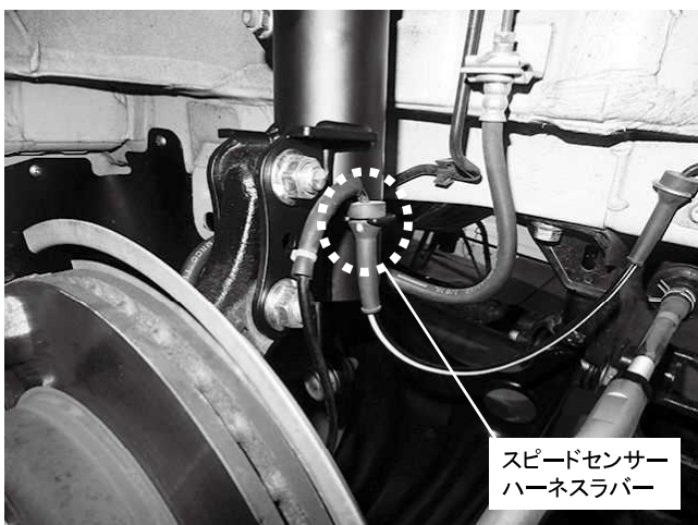
スピードセンサーハーネススラバー取り付け
