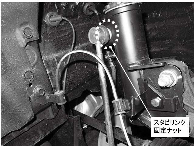
スタビリンク固定ナット 1カ所締め付け 締め付けトルク: 60\text{N}\cdot\text{m} ( 6.1\text{kgf}\cdot\text{m} ) ※スタビリングは純正品を使用してください
