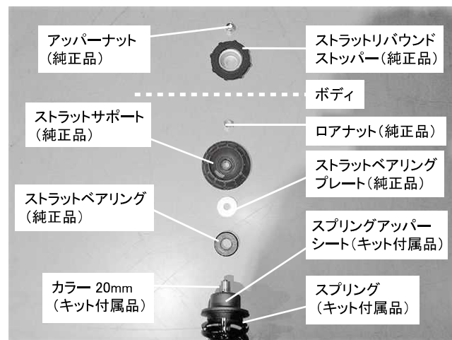
上写真を参照し、純正部品をキットに組つけてください ロアナット締め付け 締め付けトルク: 50\text{N}\cdot\text{m} ( 5.1\text{kgf}\cdot\text{m} )
