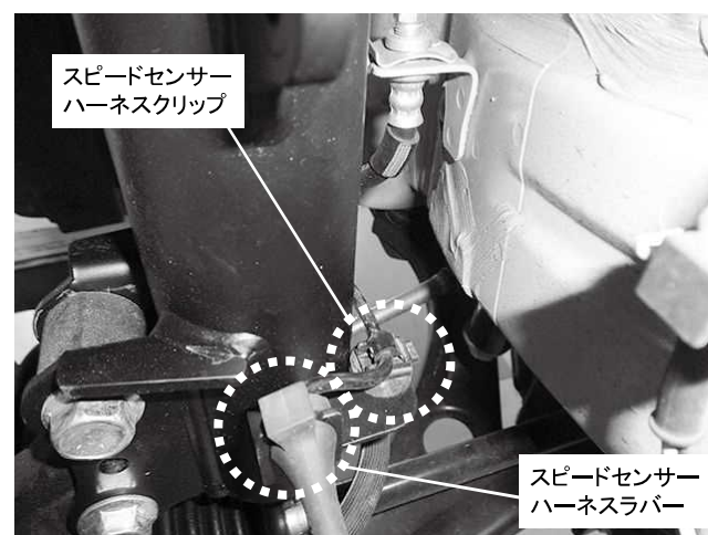
スピードセンサーハーネスクリップ 1カ所固定 ※クリップは純正品を取り外して使用してください スピードセンサーハーネ斯拉バー 1カ所固定 ※ハーネスが突っ張ってしまう場合はラバーの位置を調整してください
