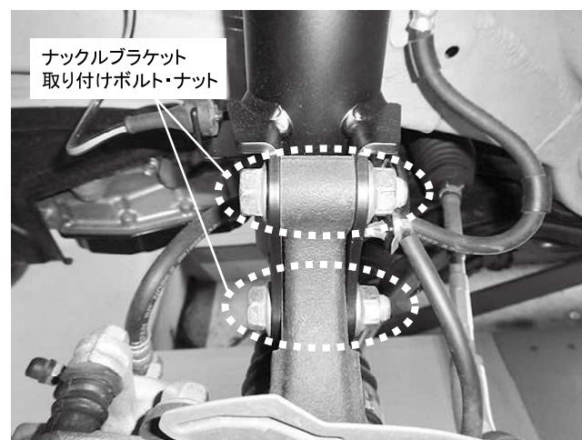
ナックルブラケット取り付けボルト・ナット 2カ所締め付け 締め付けトルク: 80\text{N}\cdot\text{m} ( 8.2\text{kgf}\cdot\text{m} )
