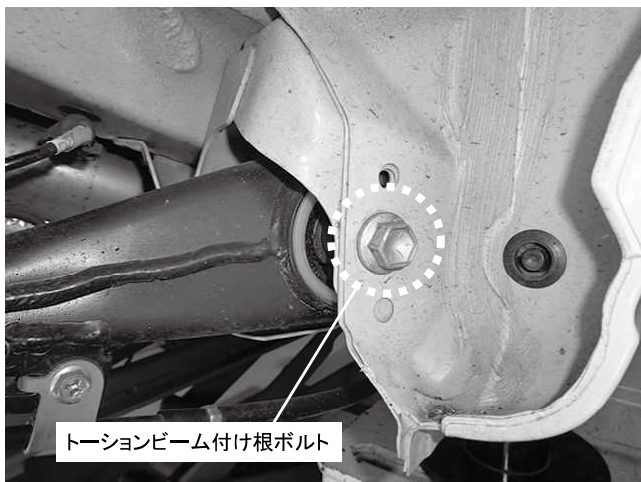
トーションビーム付け根ボルト 1カ所締め付け 締め付けトルク: 78\text{N}\cdot\text{m} ( 7.9\text{kgf}\cdot\text{m} ) ※一度緩めて1G状態で再度締め直しすることをお勧めいたします
