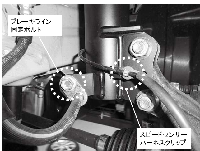
ブレーキライン固定ボルト 1カ所締め付け 締め付けトルク: 26\text{N}\cdot\text{m} ( 2.6\text{kgf}\cdot\text{m} ) スピードセンサーハーネスクリップ 1カ所固定 ※クリップは純正品を取り外して使用してください
