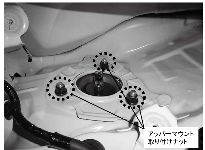
アッパーマウント取り付けナット 3カ所締め付け 締め付けトルク: 62\text{N}\cdot\text{m} ( 6.3\text{kgf}\cdot\text{m} ) ※純正ナットを使用してください
