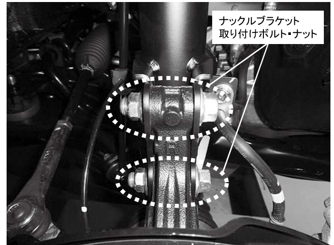
ナックルブラケット取り付けボルト・ナット 2カ所締め付け 締め付けトルク: 90\text{N}\cdot\text{m} ( 9.1\text{kgf}\cdot\text{m} ) ※取り付け上部は長穴になっておりキャンバー調整が可能です
