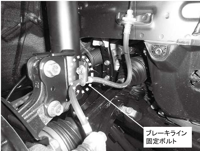
ブレーキライン固定ボルト 1カ所締め付け 締め付けトルク: 22\text{N}\cdot\text{m} ( 2.2\text{kgf}\cdot\text{m} )
