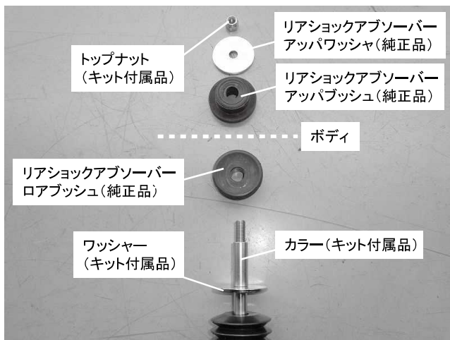
上写真を参照し、車両に取り付けてください トップナット 1カ所締め付け 締め付けトルク: 28N・m(2.9kgf・m)
