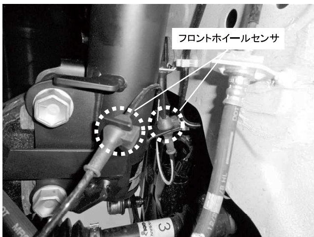
フロントホイールセンサ 2カ所取り付け ※しっかり奥まで差し込んであるか確認してください
