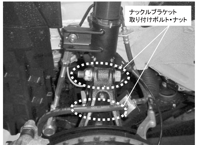
ナックルブラケット取り付けボルト・ナット 2カ所締め付け 締め付けトルク: 142\text{N}\cdot\text{m} ( 14.5\text{kgf}\cdot\text{m} ) ※ショックアブソーバーナックルブラケット上側取り付け穴は長穴になっており、キャンバー調整が可能です 左右で位置を合わせて取り付けてください
