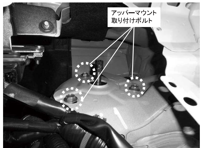
アッパーマウント取り付けボルト 3カ所締め付け 締め付けトルク: 22\text{N}\cdot\text{m} ( 2.2\text{kgf}\cdot\text{m} ) ※ボルトは純正品を使用してください ※確認車両データを確認して初めてご使用される際の推奨減衰力に合わせてください
