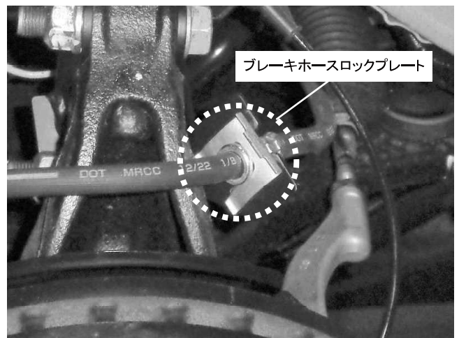
ブレーキホースロックプレート 1カ所取り付け ※しっかり奥まで差し込んであるか確認してください
