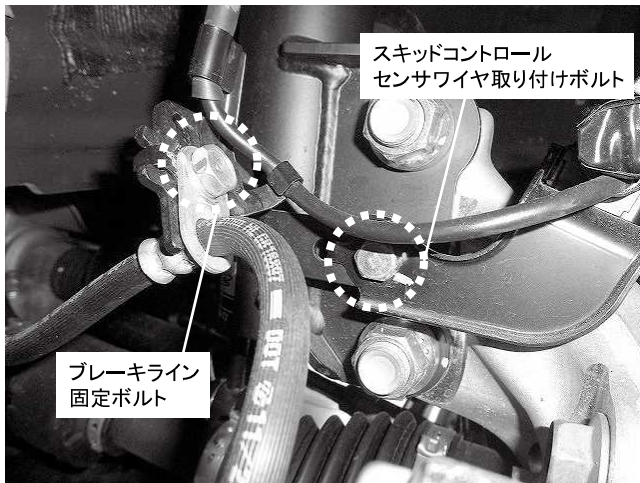
ブレーキライン固定ボルト 1カ所締め付け 締め付けトルク: 29\text{N}\cdot\text{m} ( 3.0\text{kgf}\cdot\text{m} ) スキッドコントロールセンサワイヤ取り付けボルト 1カ所締め付け 締め付けトルク: 18.8\text{N}\cdot\text{m} ( 1.9\text{kgf}\cdot\text{m} ) ※ネジ部に塗装がついて締め付けが渋い場合があります
