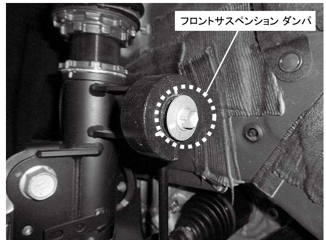
フロントサスペンション ダンパ フロントサスペンション ダンパ固定ボルト 1カ所締め付け 締め付けトルク: 20\text{N}\cdot\text{m} ( 2.0\text{kgf}\cdot\text{m} ) ※純正サスペンションより取り外して使用してください
