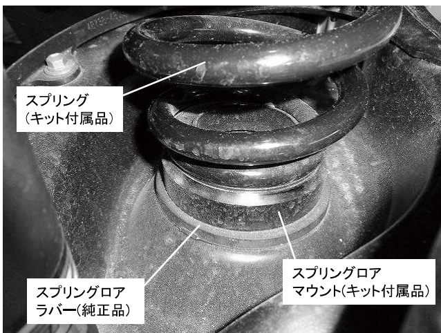
リアスプリング取り付け状態(ロア側)
