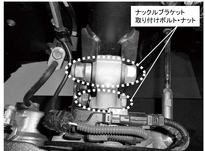
ナックルブラケット取り付けボルト・ナット 2カ所締め付け 締め付けトルク: 290\text{N}\cdot\text{m} ( 29.5\text{kgf}\cdot\text{m} ) ※ショックアブソーバーナックルブラケット上側取り付け穴は長穴になっており、キャンバー調整が可能です 左右で位置を合わせて取り付けてください
