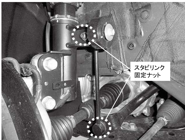
スタビリンク固定ナット 2カ所締め付け 締め付けトルク: 74\text{N}\cdot\text{m} ( 7.5\text{kgf}\cdot\text{m} ) ※CROWN CROSSOVERへ取り付ける際は、キット付属のスタビリンクを使用してください ※CROWN SPORTへ取り付ける際は、純正のスタビリンクを使用してください ※写真はCROWN CROSSOVERになります ※締め付けトルクはキット付属スタビリンク使用時も純正スタビリンク使用時も同じです
