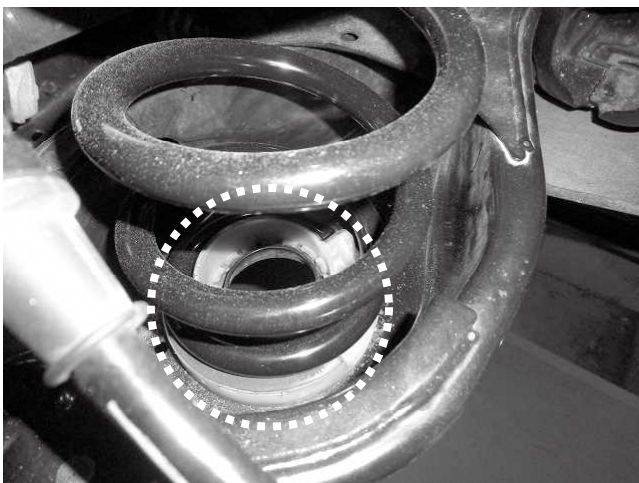
リアスプリング取り付け状態(ロア側) スプリングロアラバーがしっかりはまっているか確認してください また、スプリングの切り欠きの位置があっているかも確認してください
