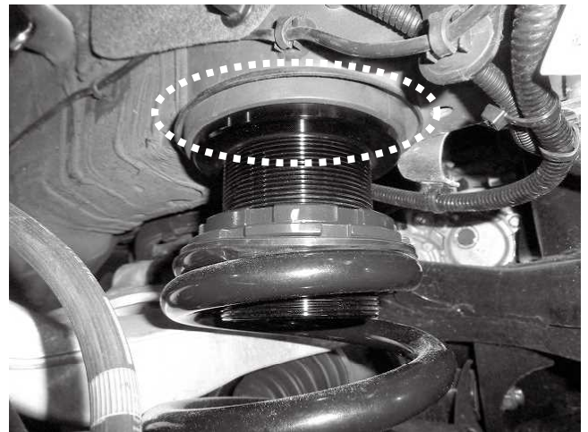
リアスプリング取り付け状態(アッパー側) スプリングアッパーラバーがしっかりはまっているか確認してください
