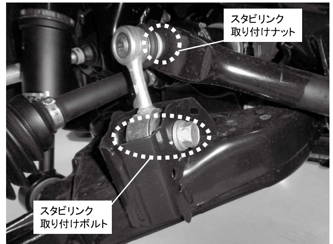
スタビリンク取り付けナット 1カ所締め付け
