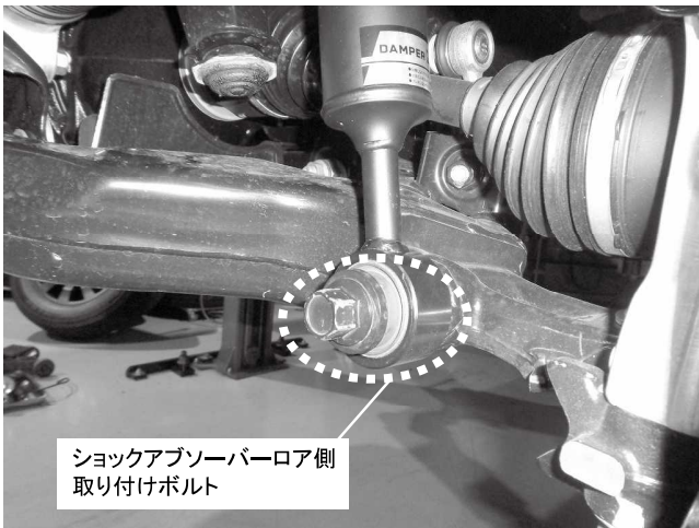
ショックアブソーバーロア側取り付けボルト
