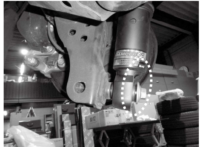
リアショックロア側取り付け状態
