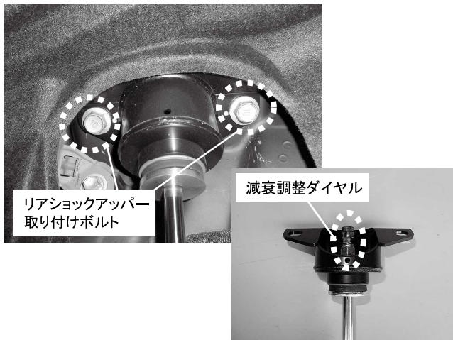
リアショックアッパータ取付けボルト 2カ所締め付け 締め付けトルク: 60\text{N}\cdot\text{m} ( 6.2\text{kgf}\cdot\text{m} ) ※減衰調整ダイヤルは構造上 アッパーマウント内部についています
