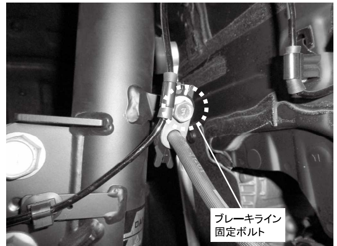
ブレーキライン固定ボルト 1カ所締め付け 締め付けトルク: 29N・m(3.0kgf・m) ※ネジ部に塗装がついて締め付けが渋い場合があります ※スピードセンサーハーネスと共締めしてあります
