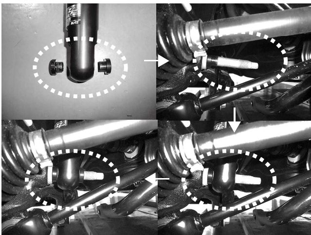
リアロアブラケット取り付けの際、そのままだと ショックとボディが干渉し取り付けにくい場合があります その際はロアブラケットからカラーを取り外して、「カラー⇒ ブラケット⇒カラー」の順に入れていくと取り付けしやすいです
