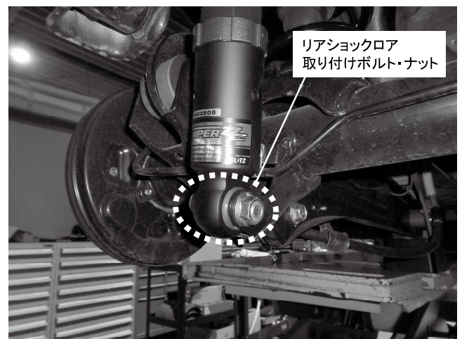
リアショックロア 取り付けボルト・ナット リアショックロア 取り付けボルト・ナット 1カ所締め付け 締め付けトルク: 80N・m(8.2kgf・m)
