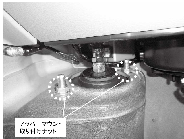
アッパーマウント 取り付けナット 2カ所締め付け 締め付けトルク: 73N・m(7.4kgf・m)
