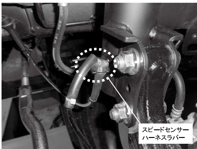
スピードセンサーハーネスラバー取り付け
