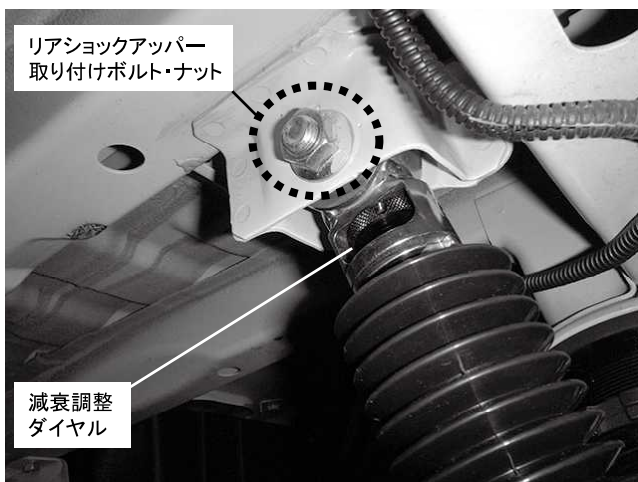
リアショックアッパー 取り付けボルト・ナット 減衰調整 ダイヤル リアショックアッパー取り付けボルト・ナット 1カ所締め付け 締め付けトルク: 80N・m(8.2kgf・m) ※減衰調整ダイヤルは構造上リアショック上部についています ※確認車両データを確認して初めてご使用される際の推奨減衰力に合わせてください
