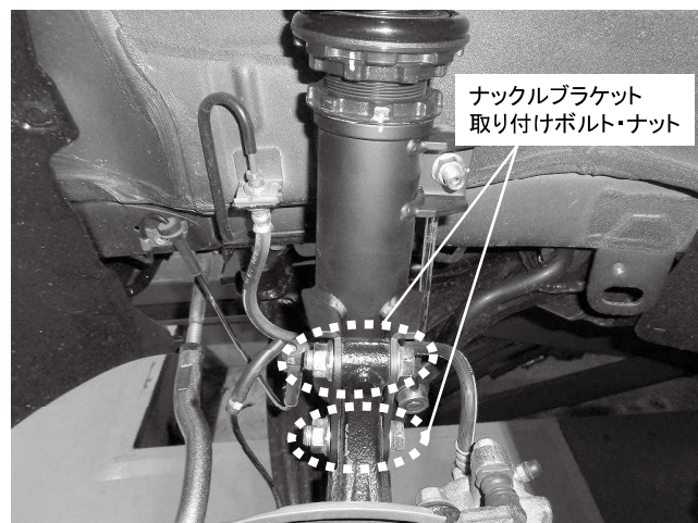
ナックルブラケット 取り付けボルト・ナット 2カ所締め付け 締め付けトルク: 95N・m(9.7kgf・m)
