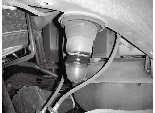
リアスプリング取り付け前に、 同梱バンブラバーを取り付けてください ※取り付け方法は別紙バンブラバー 取扱説明書を参照してください
