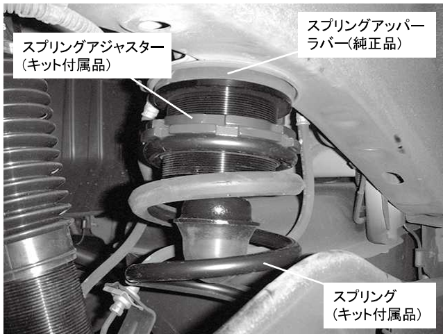
リアスプリングアッパー側取り付け状態 ※スプリングを取り付けの際、アジャスター上部に 純正スプリングアッパーラバーを取り付けてください
