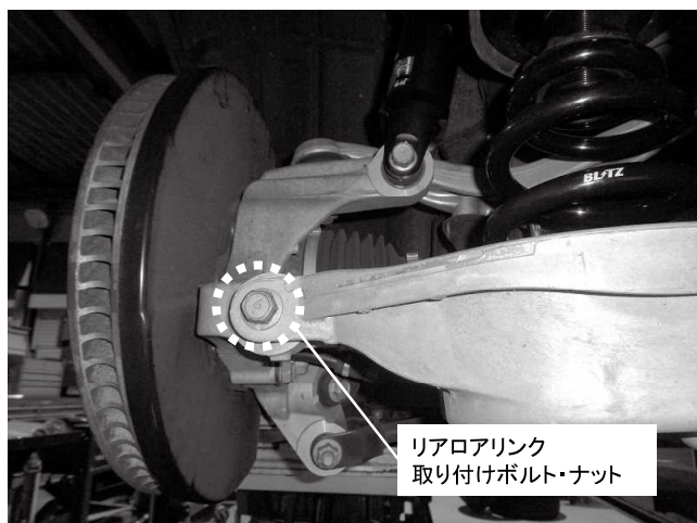
リアロアリンク取り付けボルト・ナット 1カ所締め付け 締め付けトルク: 73N・m(7.4kgf・m)
