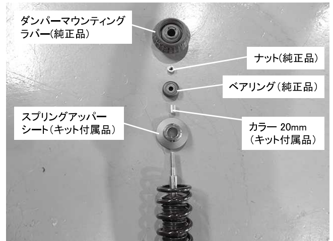
上写真を参照し、純正部品をキットに組みつけてください ベアリング固定ナット締め付け 締め付けトルク: 59\text{N}\cdot\text{m} ( 6.0\text{kgf}\cdot\text{m} )
