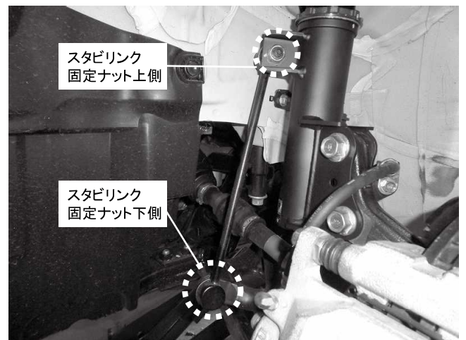
スタビリンク固定ナット上側 1カ所締め付け 締め付けトルク: 64\text{N}\cdot\text{m} ( 6.5\text{kgf}\cdot\text{m} ) スタビリンク固定ナット下側 1カ所締め付け 締め付けトルク: 38\text{N}\cdot\text{m} ( 3.9\text{kgf}\cdot\text{m} ) ※商品同梱スタビリンクを使用してください
