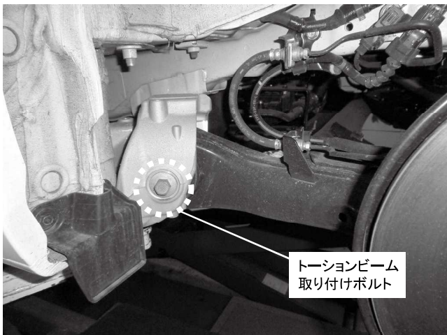
トーションビーム取り付けボルト
