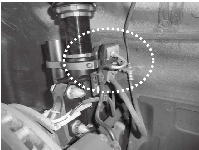
純正ブレーキライン固定ブラケットと 固定ステア、ロックシートなどとの 干渉に注意してください。
