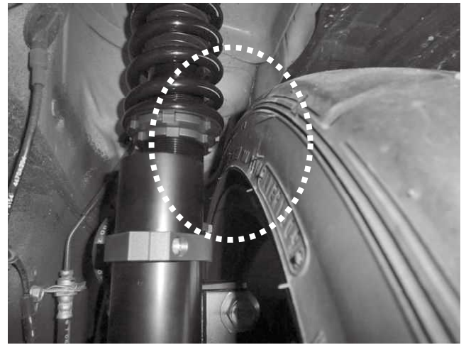
フロント タイヤ・ホイールクリアランス 18×9.5J INSET28 265/35R18装着状態 ※取り付け後クリアランス確認をお願いします。
