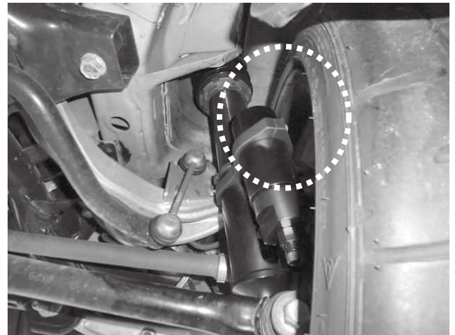
リア タイヤ・ホイールクリアランス 18×9.5J INSET28 265/35R18装着状態 ※取り付け後クリアランス確認をお願いします。
