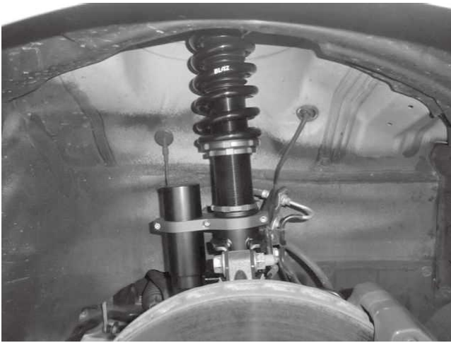
フロント右側(運転席側)取り付け状態
