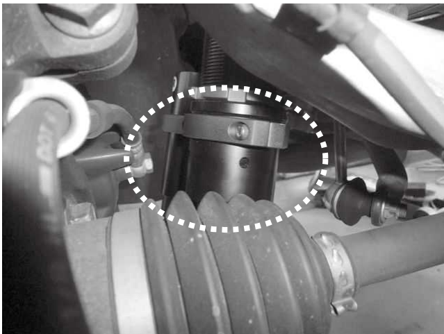
リザーバータンク固定ステーとドライブシャフト ブーツとの干渉に注意してください。
