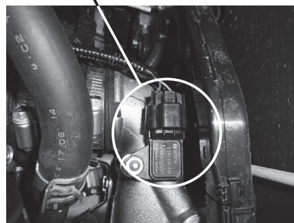
サブ側圧力センサー
