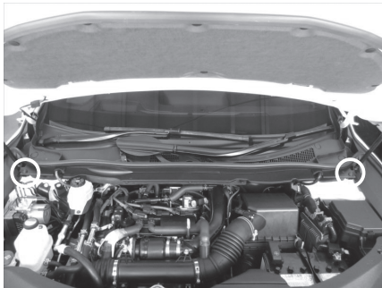
ワイパーアーム ボルト 3 カ所 カウル クリップ 2 カ所（丸部）
