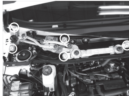
ワイパーリンク ボルト 5 カ所（丸部） コネクター 1 カ所
