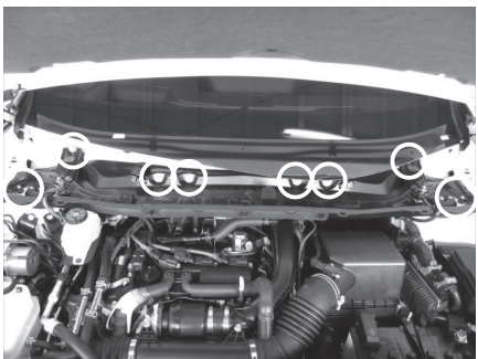
プレート ボルト 6 カ所（丸部） ナット 6 カ所（丸部）
