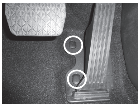
カバーを外し、ボルト2本を取り外す。
