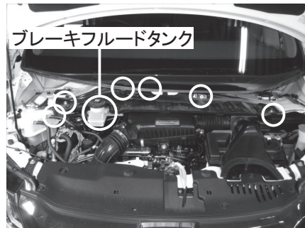
ブレーキフルードタンク ボルト 2 カ所 プレート ボルト 6 カ所（丸部）
