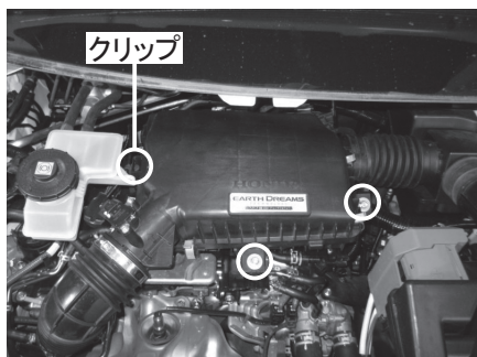
クリップ ボルト 2 カ所（丸部）、クリップ 1 カ所 エアフロセンサー、ダクト 2 カ所 グロメット 1 カ所
