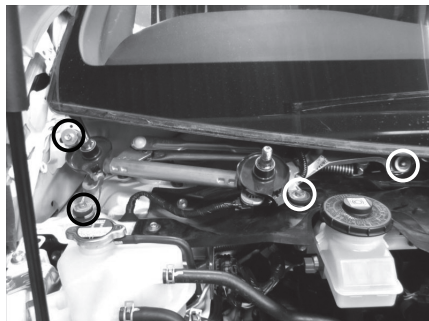
ワイパーリンク ボルト 4 カ所（丸部） コネクター 1 カ所
