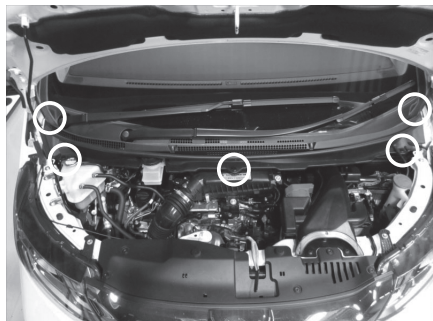
ワイパーアーム ボルト 2 カ所 カウル部 クリップ 5 カ所（丸部）
