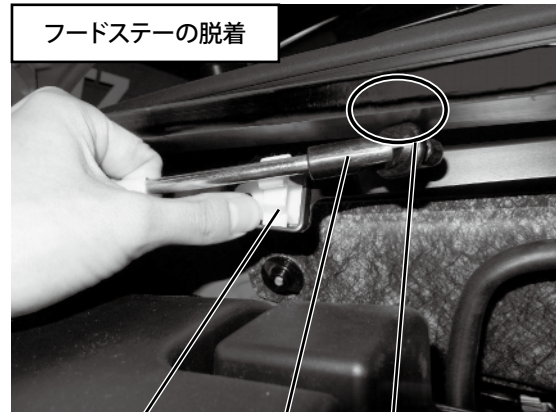
フードステーの脱着 フードステークランプ フードステー クリアランス確認箇所 タワーバーシャフトとフードステーとの クリアランス約3mm
