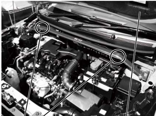
ボンネットインシュレーター クリアランス確認箇所 タワーバーシャフトとボンネットインシュレーターとの クリアランス約11mm
