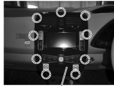
クラスターリッドC かん合
