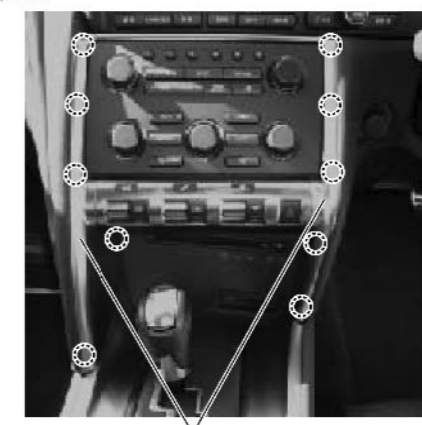
インストールガーニッシュ ○かん合
