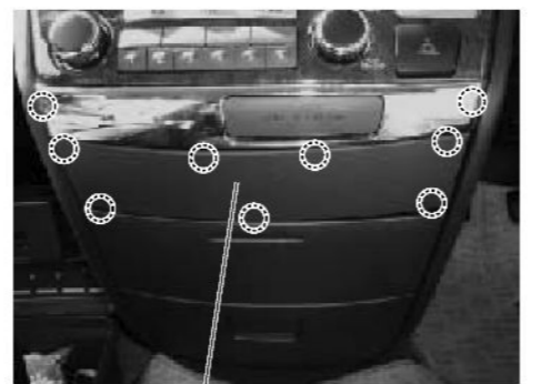
クラスターリッドセンターロア ○かん合
