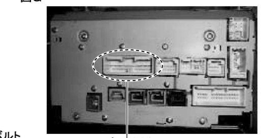
26ピンコネクタ
