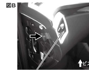
サイドベンチレーターフィニッシャーB(L)
