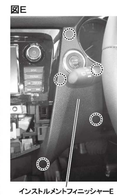
かん合 インストルメントフィニッシャーE
