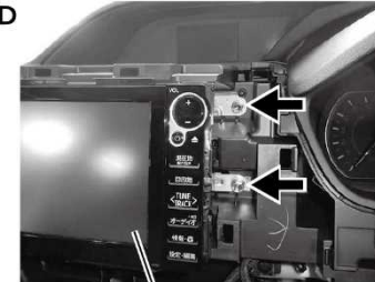
TVモニターASSY
