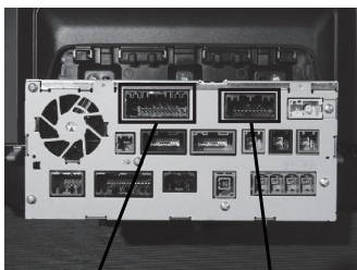
24ピンコネクタ 20ピンコネクタ
