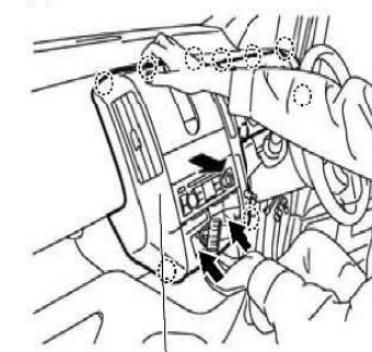
クラスターリッド ○かん合 ↑ネジ
