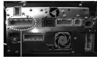
40ピンコネクター
