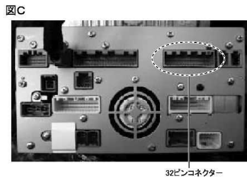
32ピンコネクター
