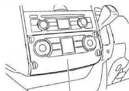
かん合 フロントコントローラー
