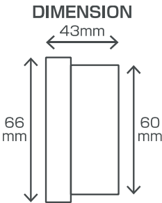
Meter Dimension
